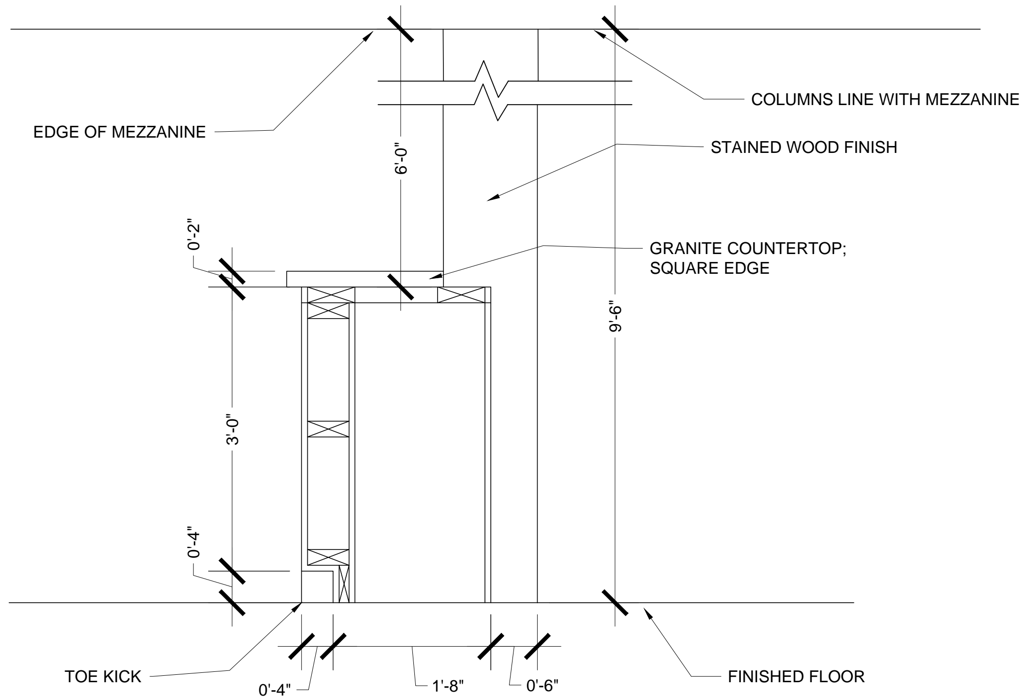
① SECTION PLAN SCALE: 0'-1" = 1'-0"
